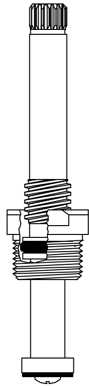
403601 403602 18 Threads per Inch Gland
